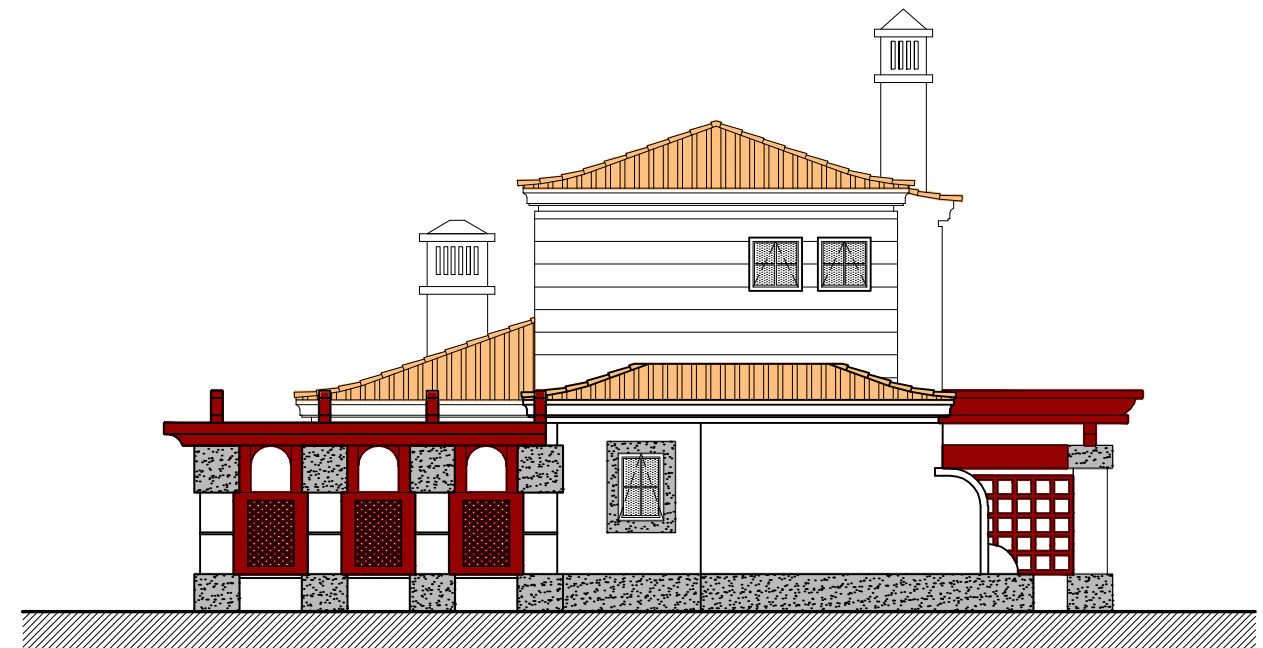
ALÇADO LAT.DIREITO
