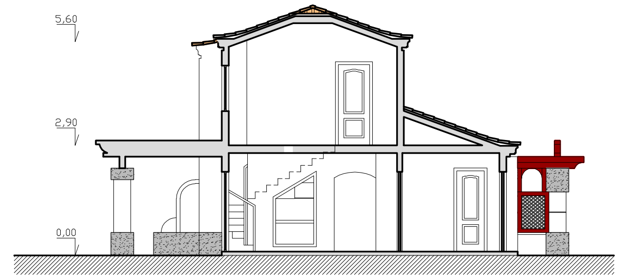
CORTE AB
